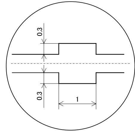
ストップパー部詳細図 Detail of stopper
