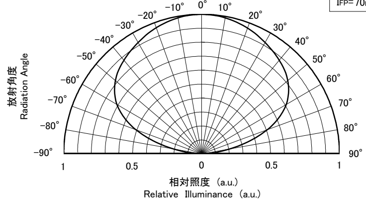
■ 指向特性 Directivity Ta=25°C IfP=70mA
