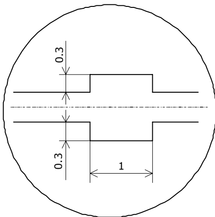
ストップ部詳細図 Lead Standoff
