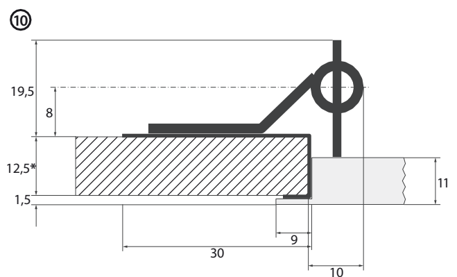
Alle Maße in mm *gesonderte Einbausätze für größere Deckenstärken erhältlich
